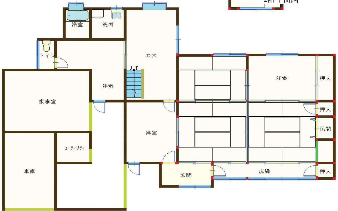
2階平面図
