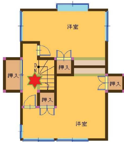
2階平面図
