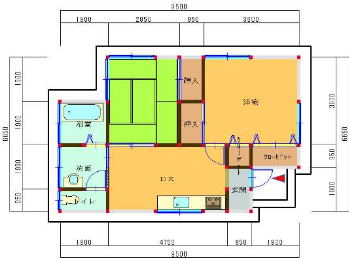
1階平面図
