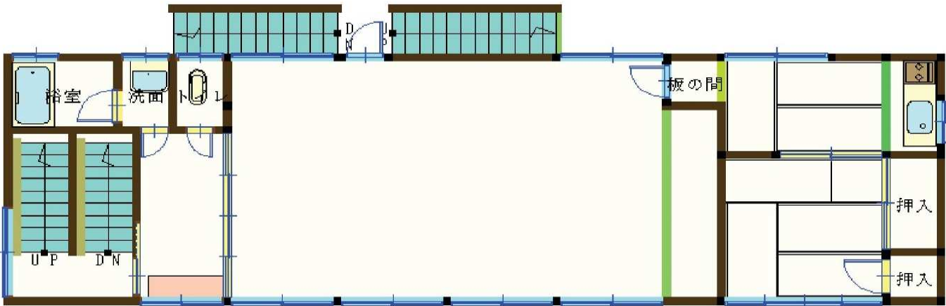
2階平面図
