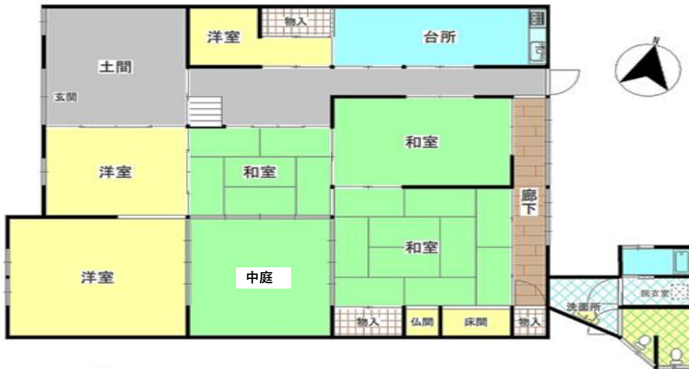
1階平面図
