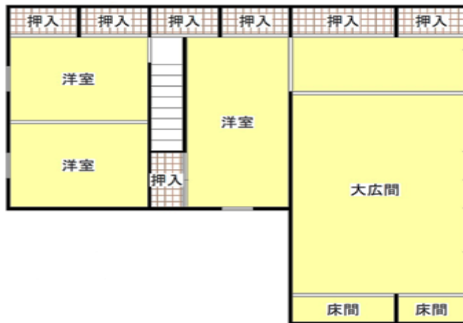
2階平面図
