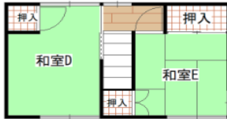
2階平面図
