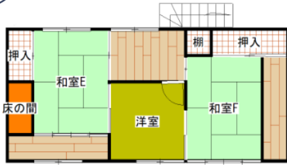
2階平面図
