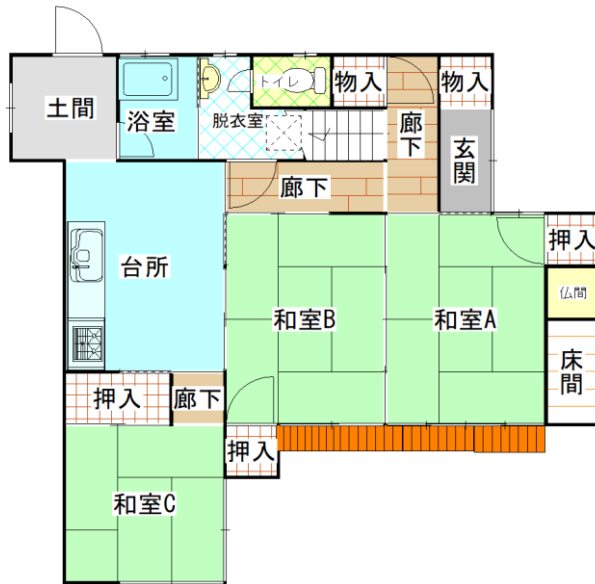
1階平面図
