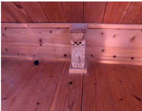
2階梁接合部
