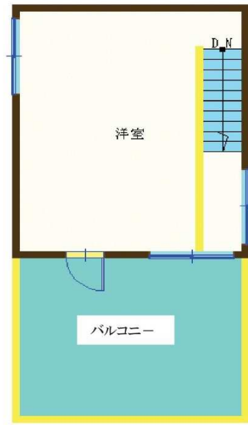
2階平面図
