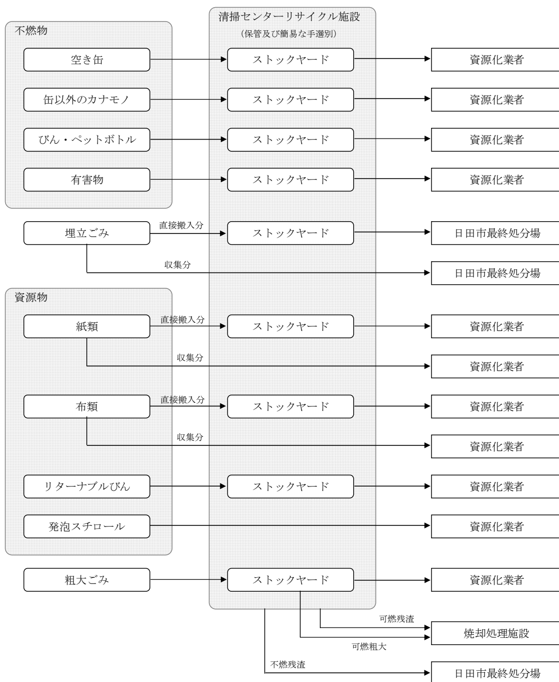
図 9-3 現有施設における不燃物、埋立ごみ、資源物等の流れ
