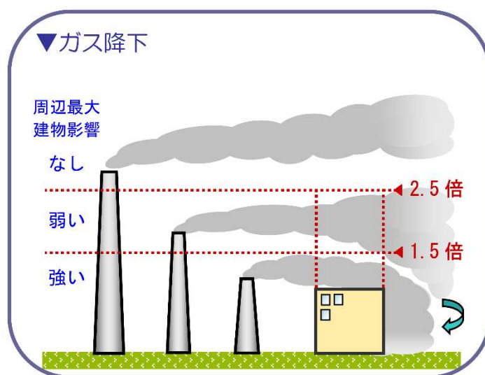
図 8-3 ダウンドラフト現象
