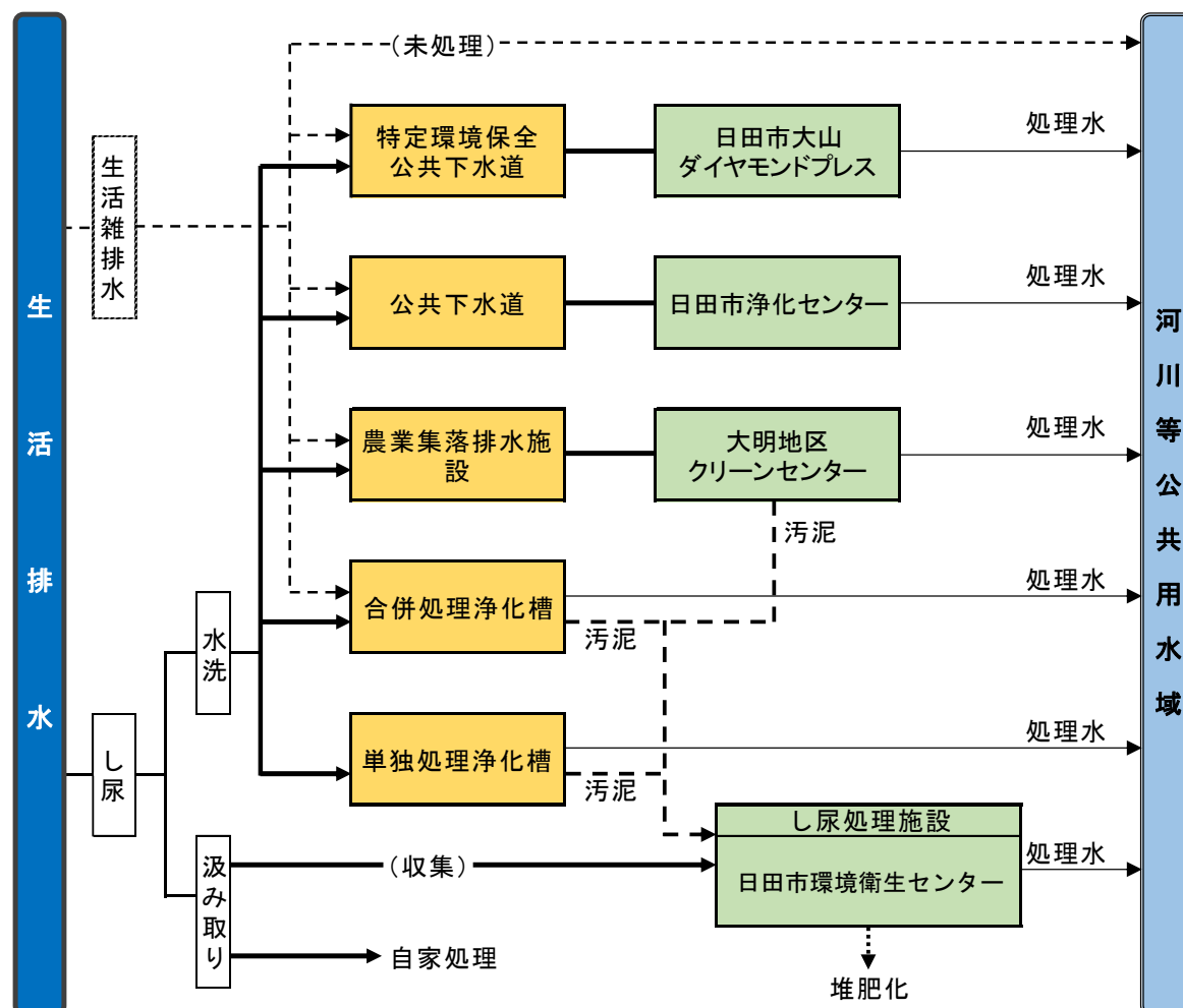
図 4-1-2 生活排水処理体系（令和 6 年 3 月末現在）
