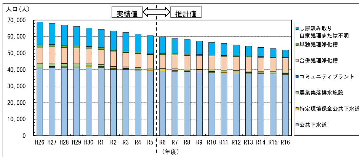
図 4-2-2 処理形態別人口の将来予測の結果（目標達成時）
