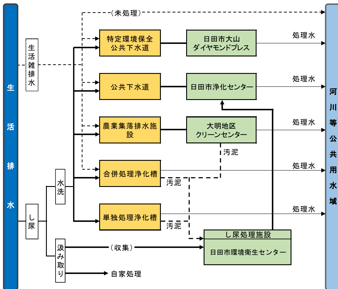
図 4-2-1 生活排水処理体系（目指す姿）
