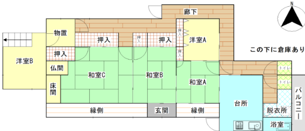
1階平面図
