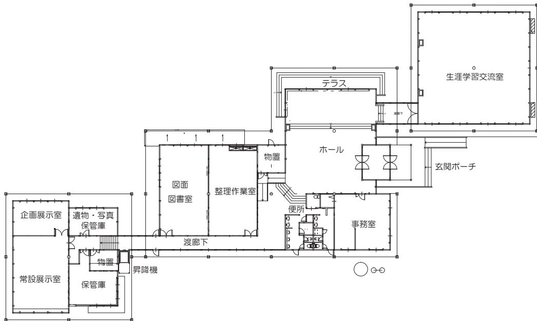
埋蔵文化財センター平面図
