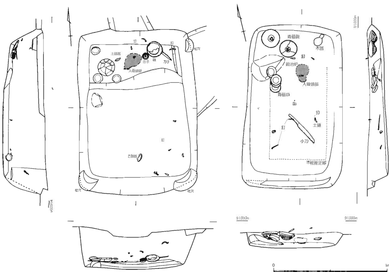
C区下層2号 (左)・4号 (右) 中世墓実測図 (1/20)
