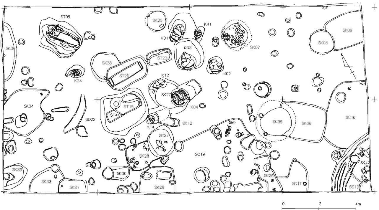
吹上遺跡第9次B地点遺構配置図 (1/120)
