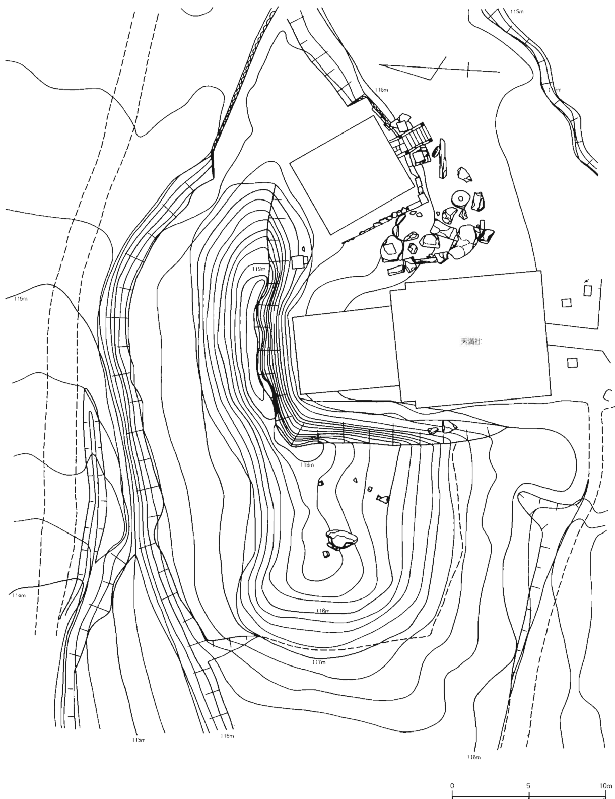
天満1号墳墳丘測量図 (1/250)
