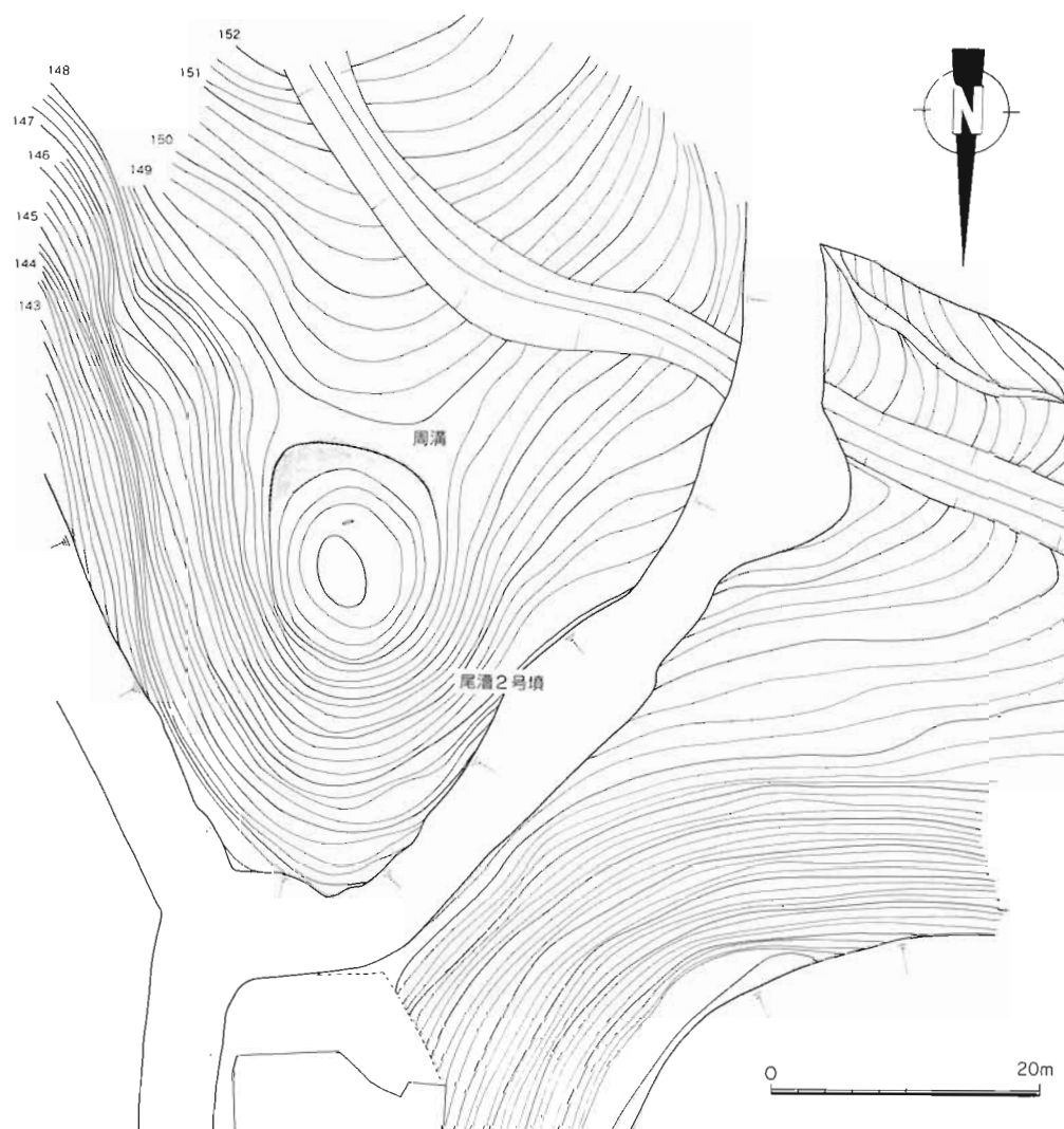
尾澗2号墳周辺地形測量図 (1/600)
