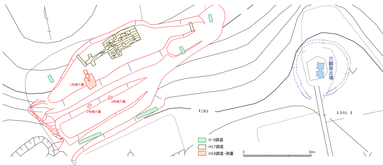
調査区配置図 (1/1,000)
