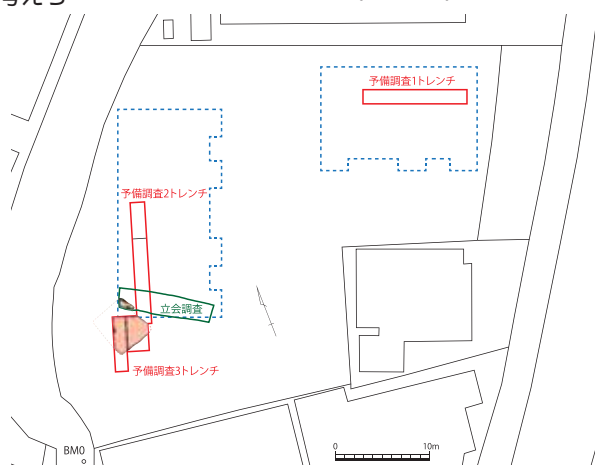
トレンチ配置図 (1/800)
