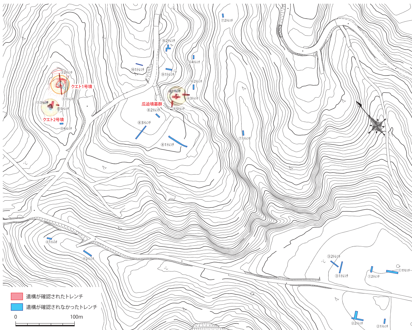
トレンチ配置図 (1/2,000)
