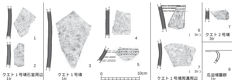
クエト1・2号墳、瓜迫墳墓群出土土器実測図(1/6)
