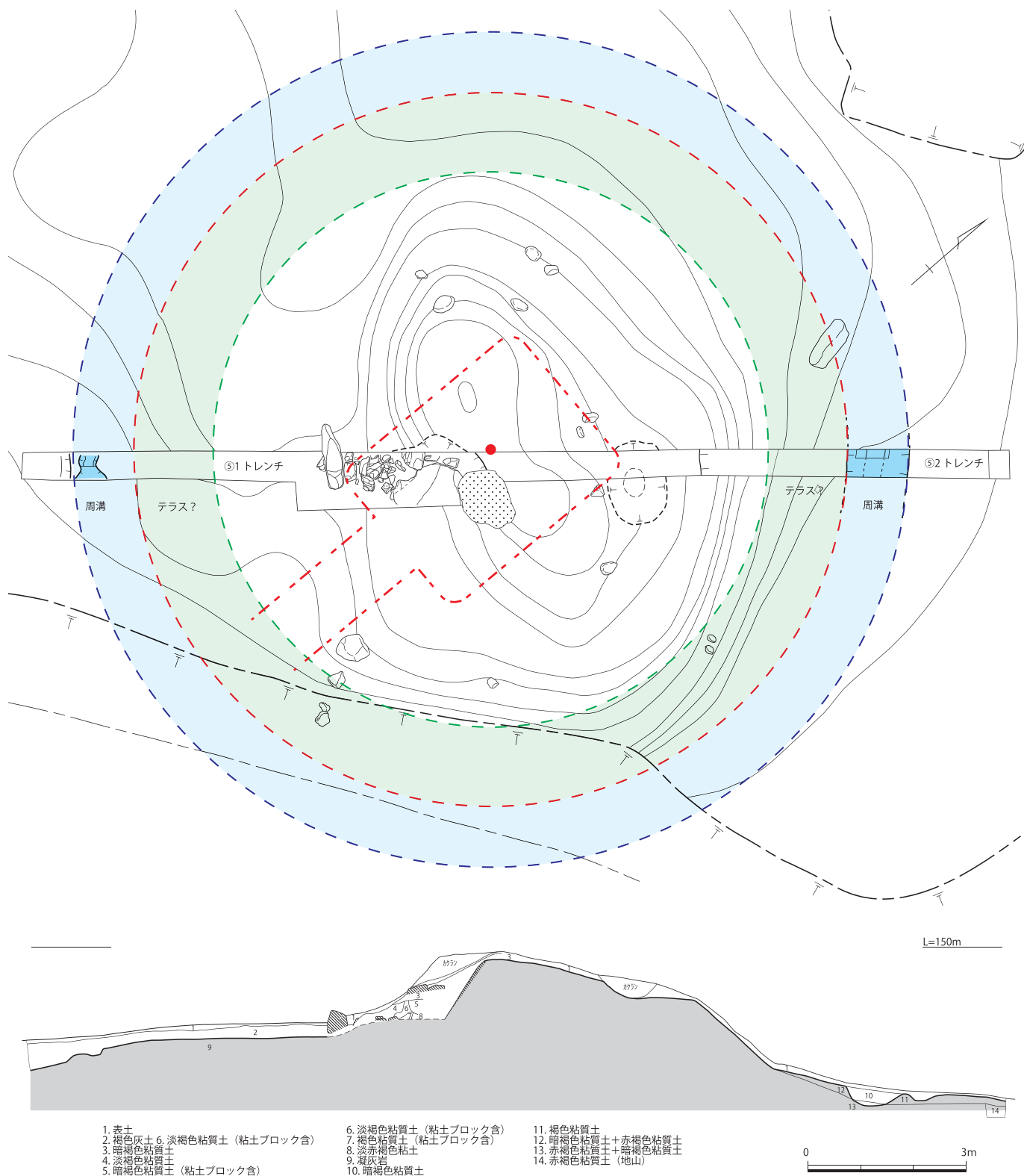
クエト 1 号墳測量図 (1/110)
