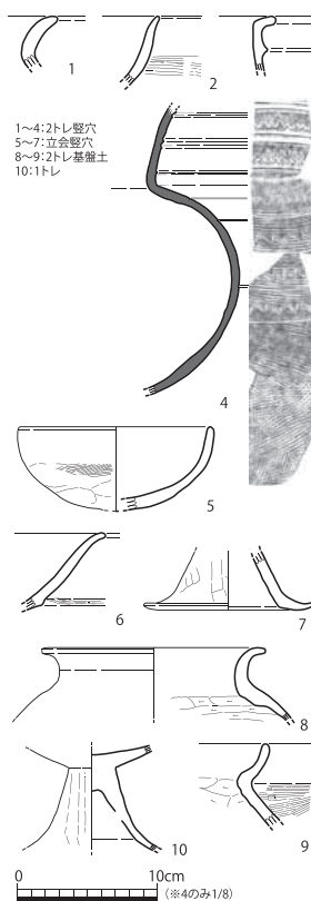
出土遺物実測図 (1/6)
