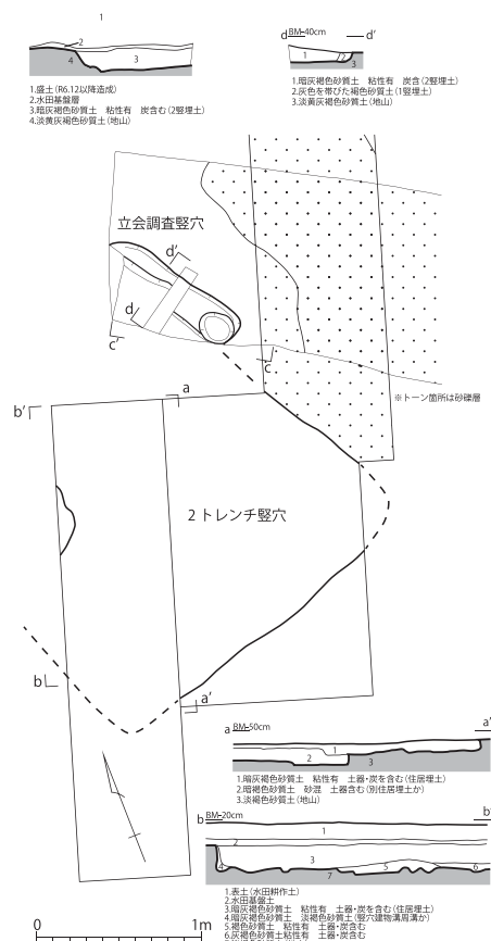
竪穴建物実測図 (1/50)
