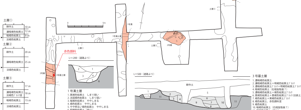
遺構配置図 (1/300)
