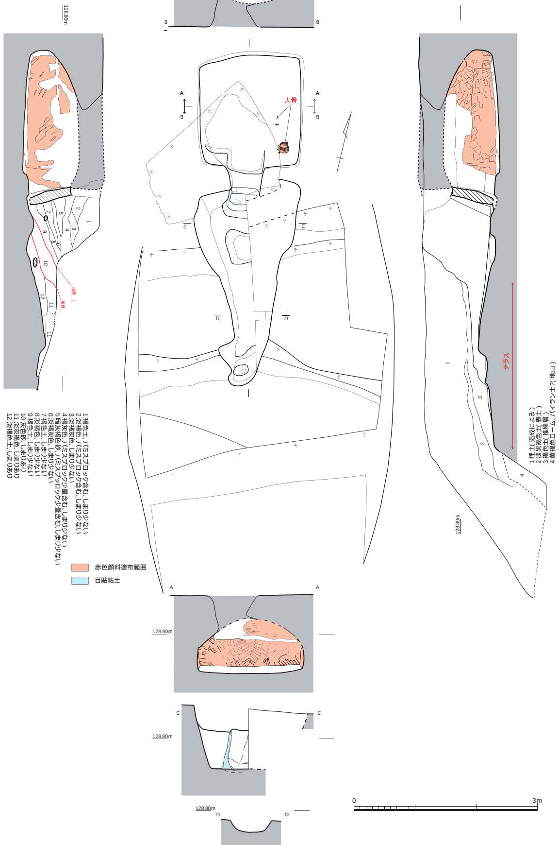
1 号横穴墓実測図 (1/60)
