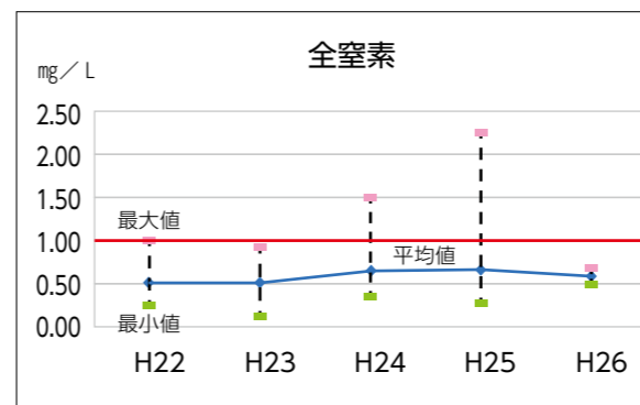
全窒素
