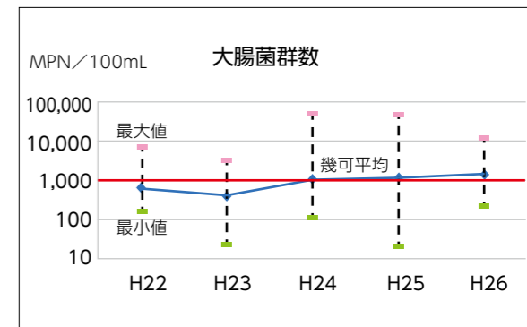
大腸菌群数
