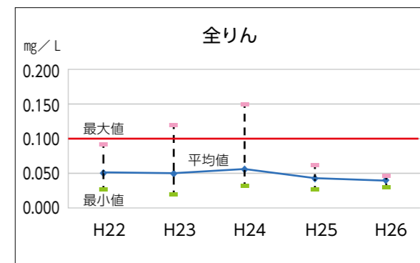
全りん
