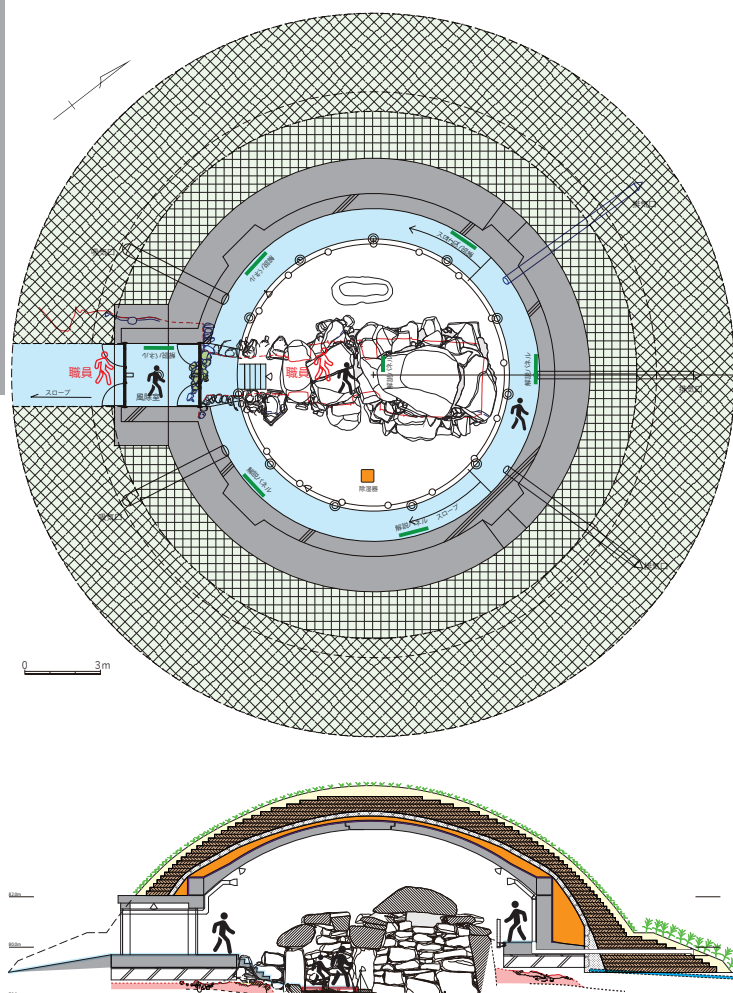
1 号墳保存施設（1/300）
